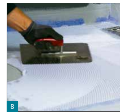
8 Die erste Lage mit einem 4 mm Zahnglätter aufkämmen und anschließend glätten.
